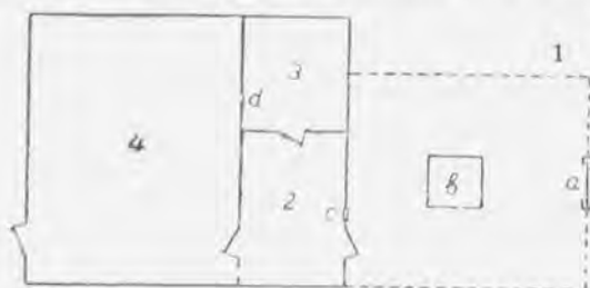
План песцовой кормушки-ловушки:
